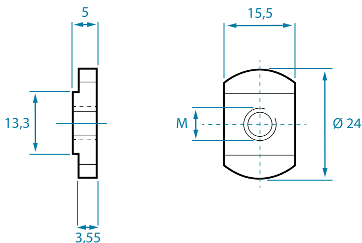
Écrou pour rail sans ressort
